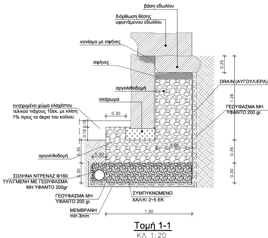
Σχέδιο 2. Τομή 1-1 (Απόσπασμα από την Υπ' αριθμ. πρωτ: ΥΠΠΟΑ/ΓΔΑΜΤΕ/ΔΑΑΜ/ΤΜΑΜ/313471/32418/938/344/23-07-2018 (ΑΔΑ: ΩΣΖ04653Π4-8ΞΒ) Υ.Α. εγκεκριμένη μελέτη «Μελέτη αποκατάστασης του αρχαίου θεάτρου της Λάρισας»)
